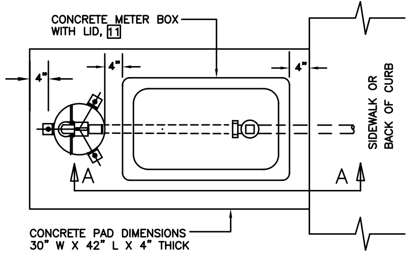
PLAN N.T.S.
